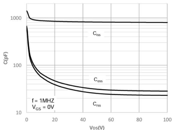
Capacitance - V_{DS}
