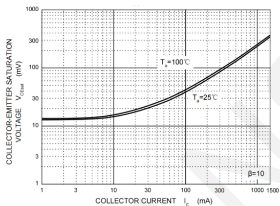
V_{CEsat} \sim I_C
