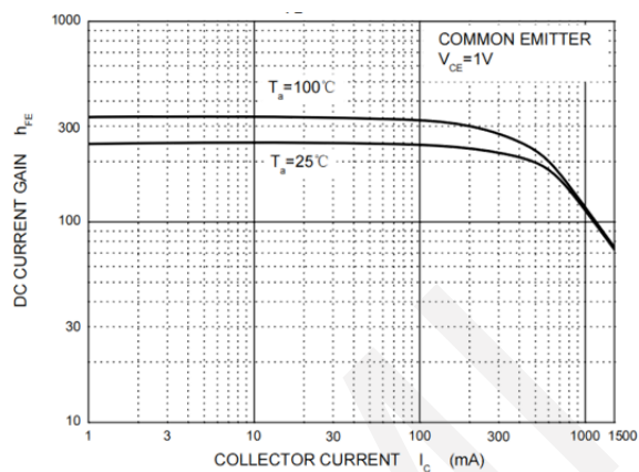
h_{FE} \sim I_C
