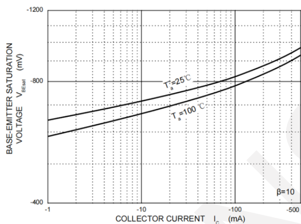
V_{BE(sat)} \sim I_C
